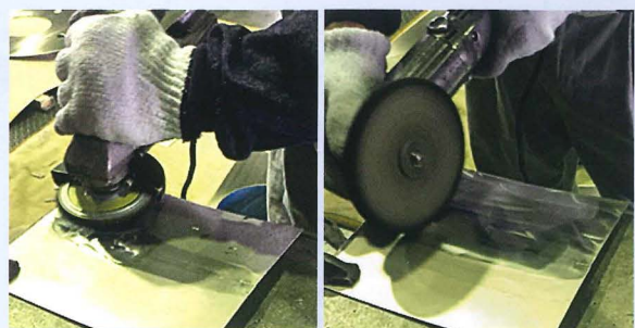
研磨剤
